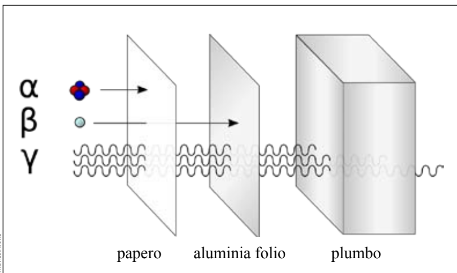
La bildo montras eblon de tri specoj de radioaktiveco penetri materialojn. Alfa-radiadon (α) eblas haltigi per folio de papero, beta-radiadon (β) - per aluminia folio. Por haltigi gama-radiadon (γ) bezonatas kelkcentimetra tavolo de plumbo.
